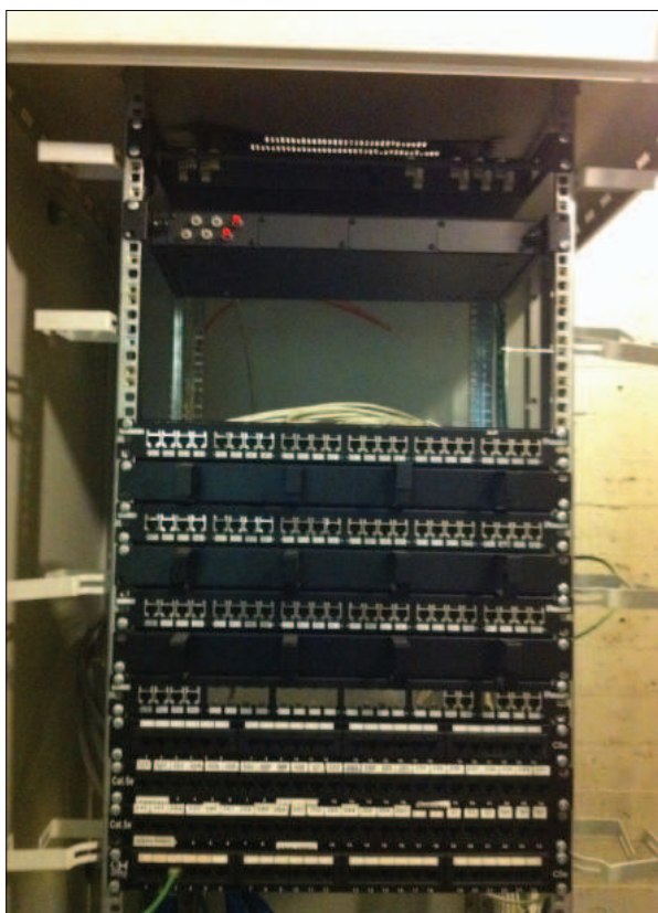
Posa cavi in fibre ottiche e cavi utp per cablaggio strutturato per il nuovo capanone. Armadio generale dati e controllo video-camere
