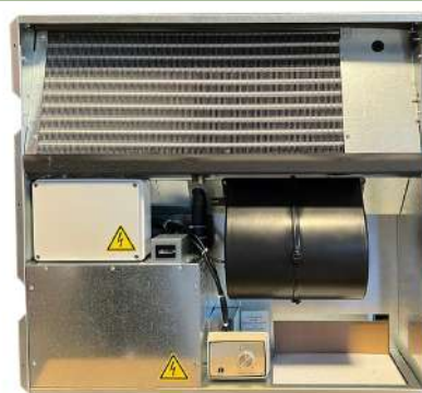
Macchina completa
