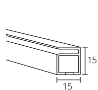
153200 Profilo Profile Profil
