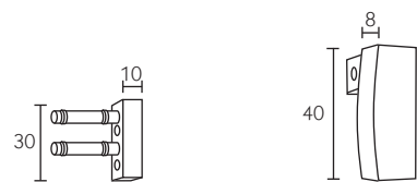
313045 423101 Tappo Endkappe Endcap Tapón Bouchon Zatyczka
