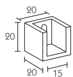
153001 Rosetta a muro Recess bracket Naissance murale
