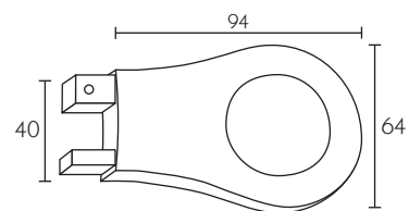
423026 Terminale Endstück Fial Terminal Embout Końcówka
