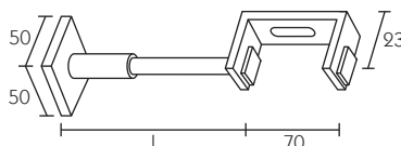
3134-- Supporto doppio Double bracket Support double
