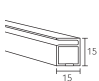
153200 Profilo Profile Profil
