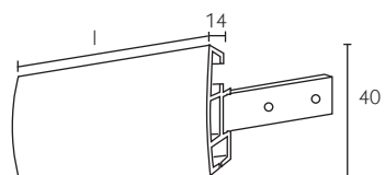
423007 Angolo Angle Retour
