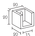
153001 Rosetta a muro Recess bracket Naissance murale
