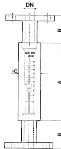
Attacco assiale flangiato
