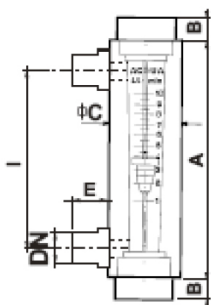
Attacco assiale filettato
