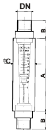
Attacco assiale filettato
